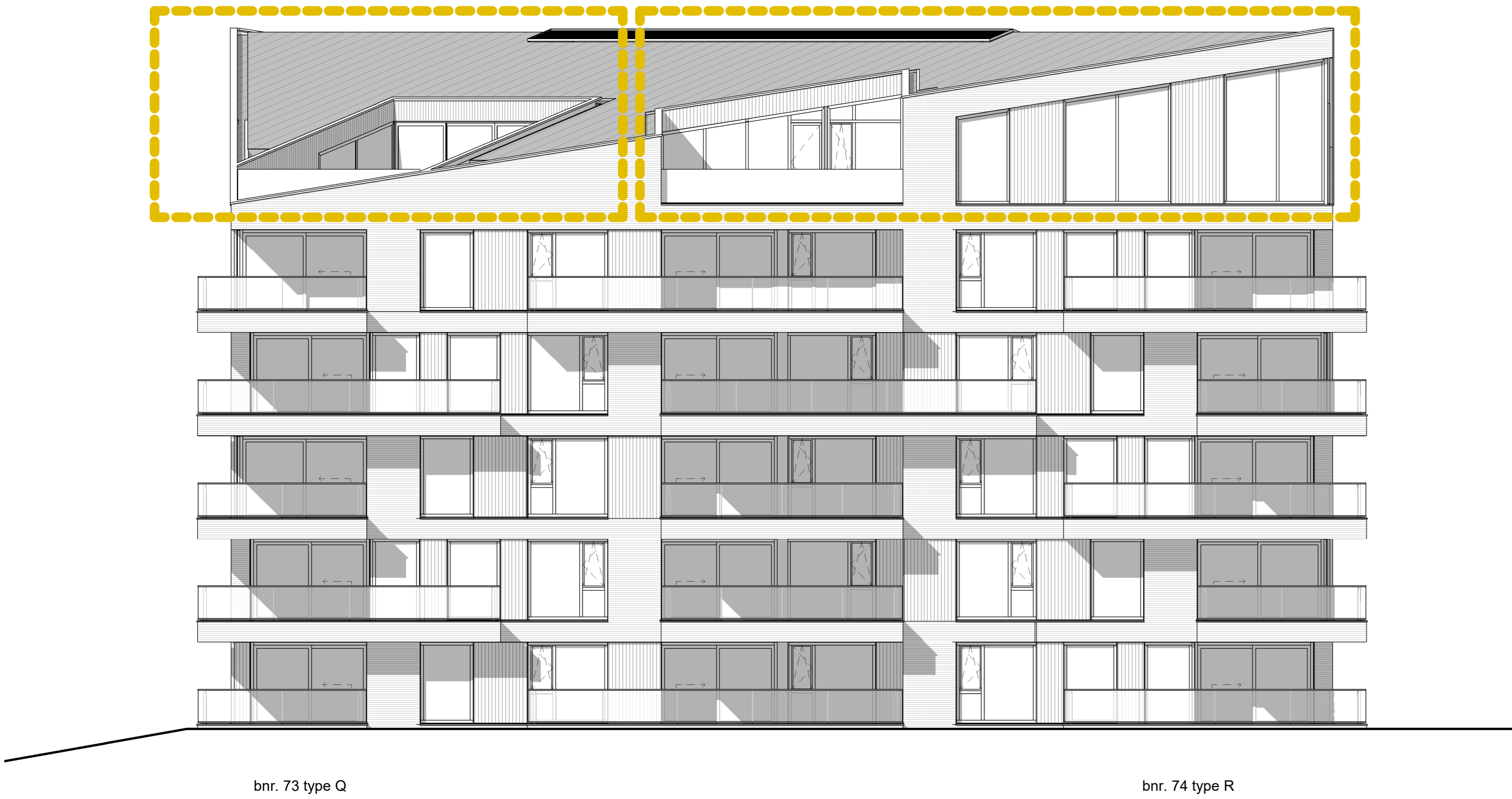
Voorgevel 1:100
