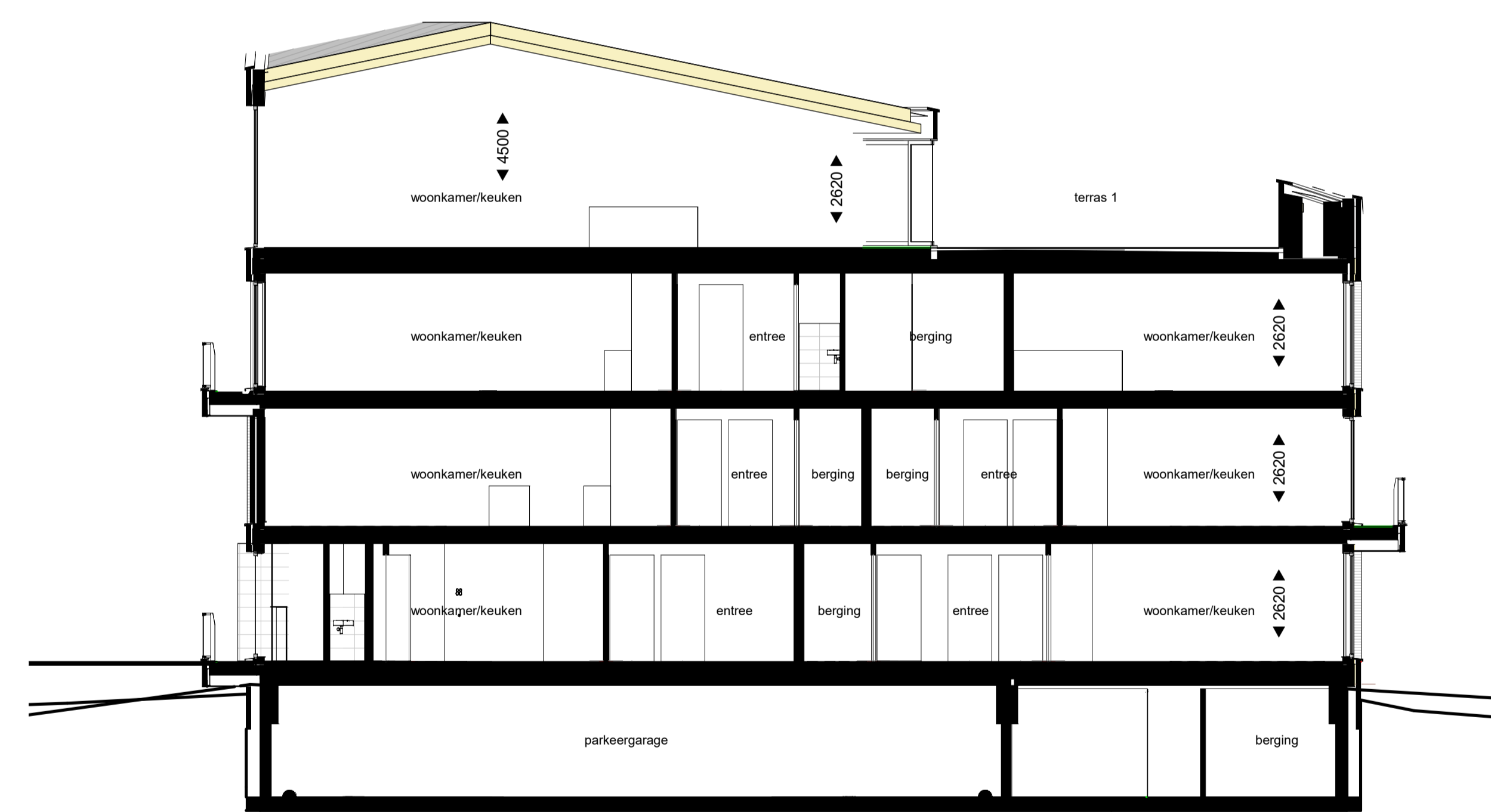
Doorsnede gebouw A 1 : 100
